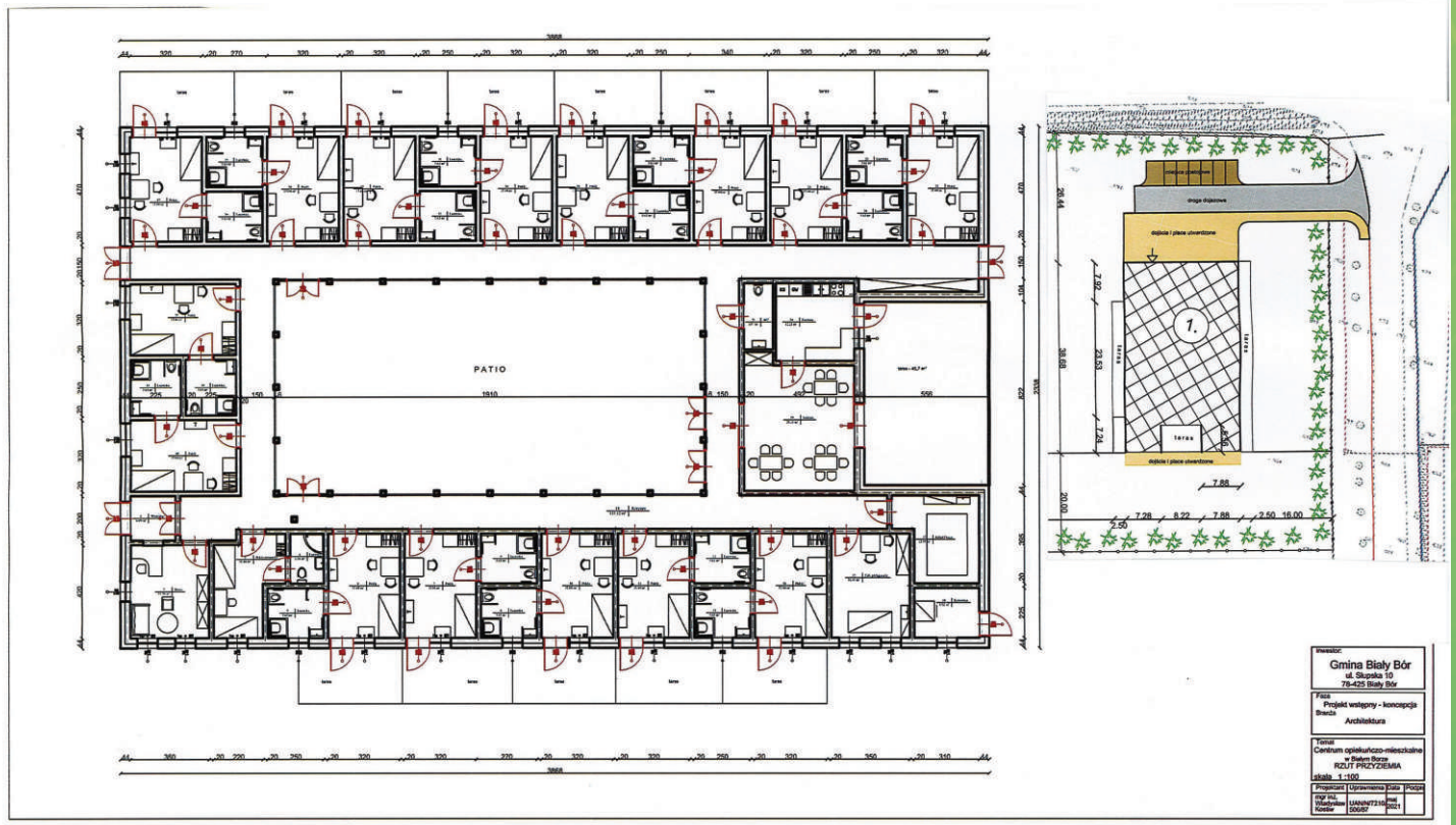
Projekt Centrum Opiekuńczo-Mieszkaniowego w Białym Borze
